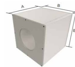
Variante 1: Wanddurchführung mit Rauchrohrausschnitt DN 130 bis DN 200
